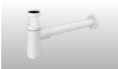
KC32SIRU-MW matt weiß Design Siphon, rund Massiv aus Messing Tauchrohr 8,5 cm / Wandrohr 30 cm
