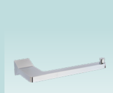
WC-Papierhalter KCA1003C Gewicht: 360 g Maße: 168 x 28 x 70 mm
