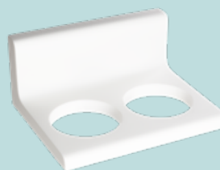
Wandhalter KCMA011W passt zu Seifenspender KCMA012W und Zahnputzbecher KCMA013W Wandmontage, inkl. Montageset weiß, 150 x 120 x 65 mm
